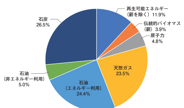
図-2 世界のエネルギー供給
