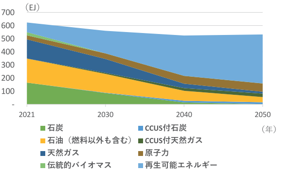
図-1 ネットゼロ排出シナリオ・エネルギー供給予測
